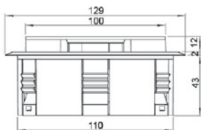
Easy-Outlet-TA zum Ausführen einzelner Kabel
