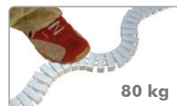
Trittfest Trittfestigkeit gestreckt bis 80 kg zusammengeschoben bis 100 kg
