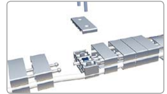
Easy-Stop Zugentlastung für bis zu 16 Kabel
